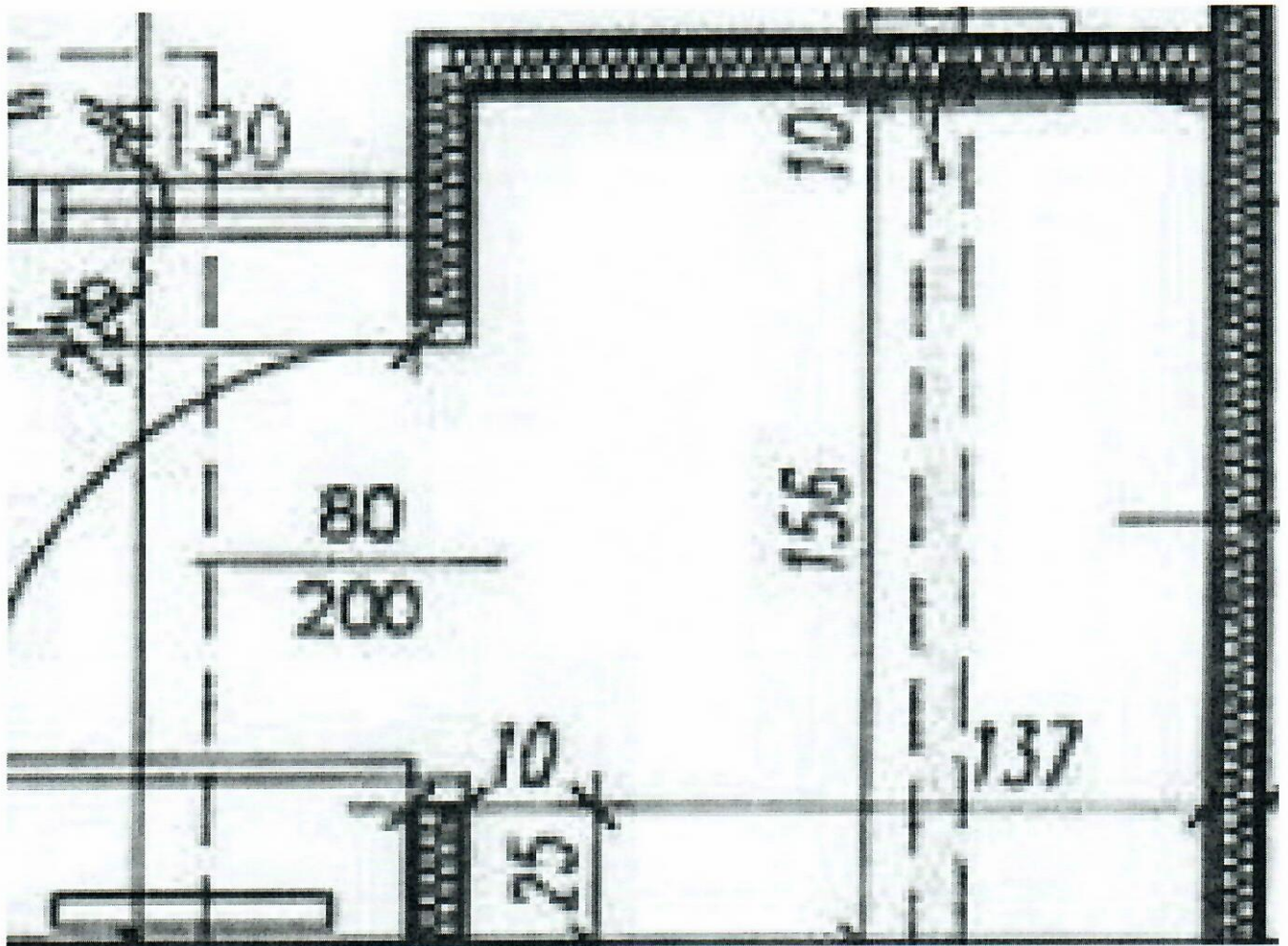
Schemat 2 - (wysokość pomieszczenia ok. 2,5m) – 2,14m 2 ok. (137x156)
